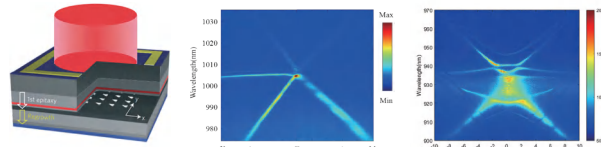
光子晶体激光器 (PCSEL) 的荧光特性
