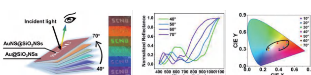
结构色角度依赖性表征
