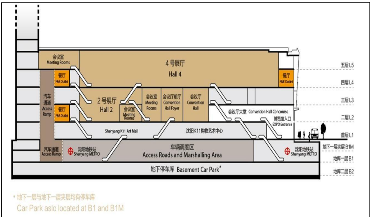
博览馆楼层示意图
