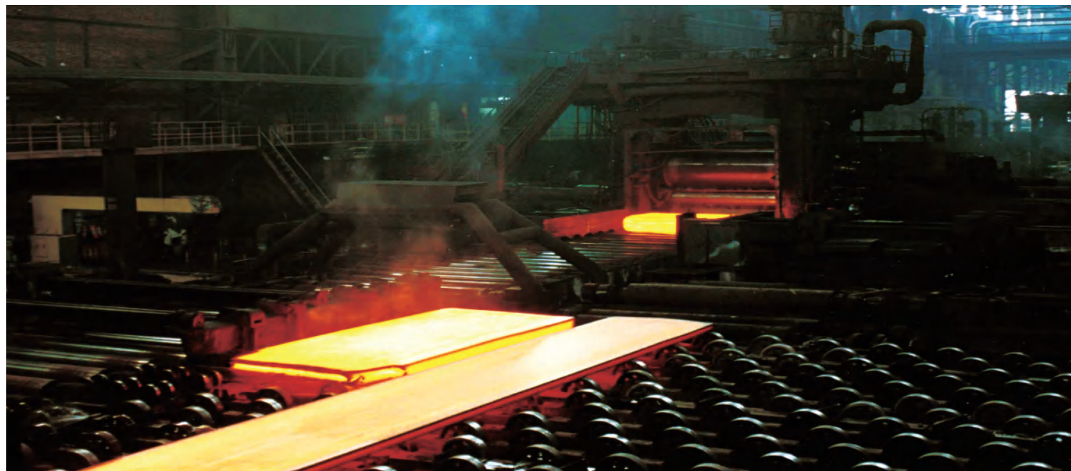
舞阳钢铁有限责任公司4200mm热轧生产线 Wuyang Iron & Steel Co., LTD. 4200mm hot rolling production line
