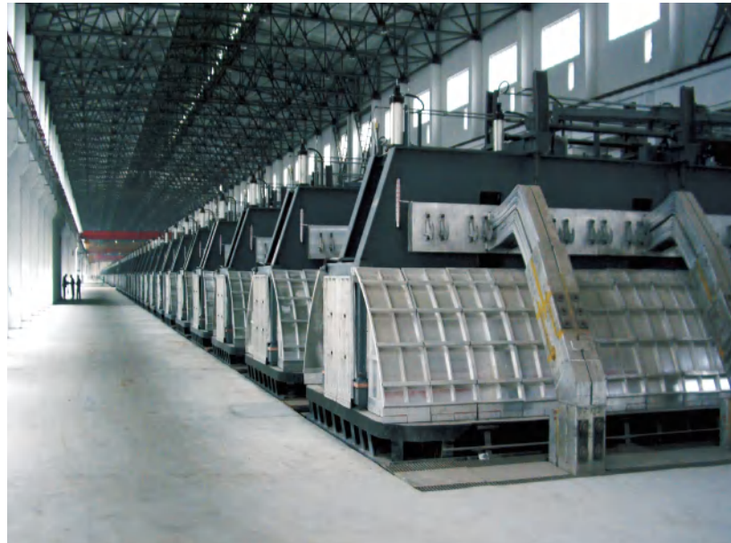
云南文山铝业500KA电解铝项目 Yunnan Wenshan Aluminum 500KA Electrolytic aluminum project
